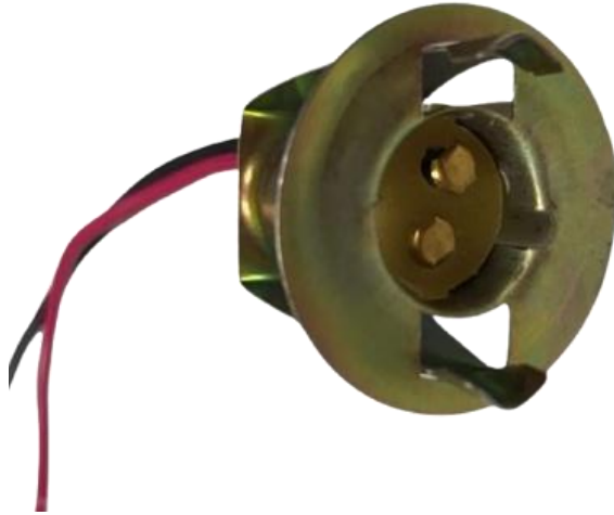
65-024 Arnés Socket Universal 2 Polos R10W
